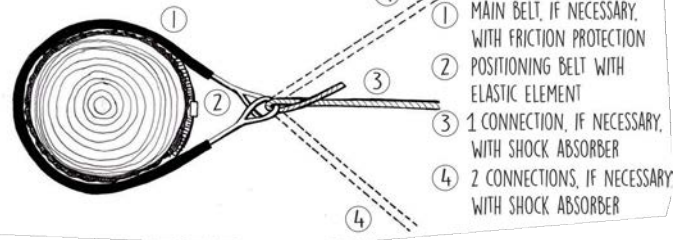
Figuur 9: Bevestiging van een uit meerdere componenten bestaand systeem
